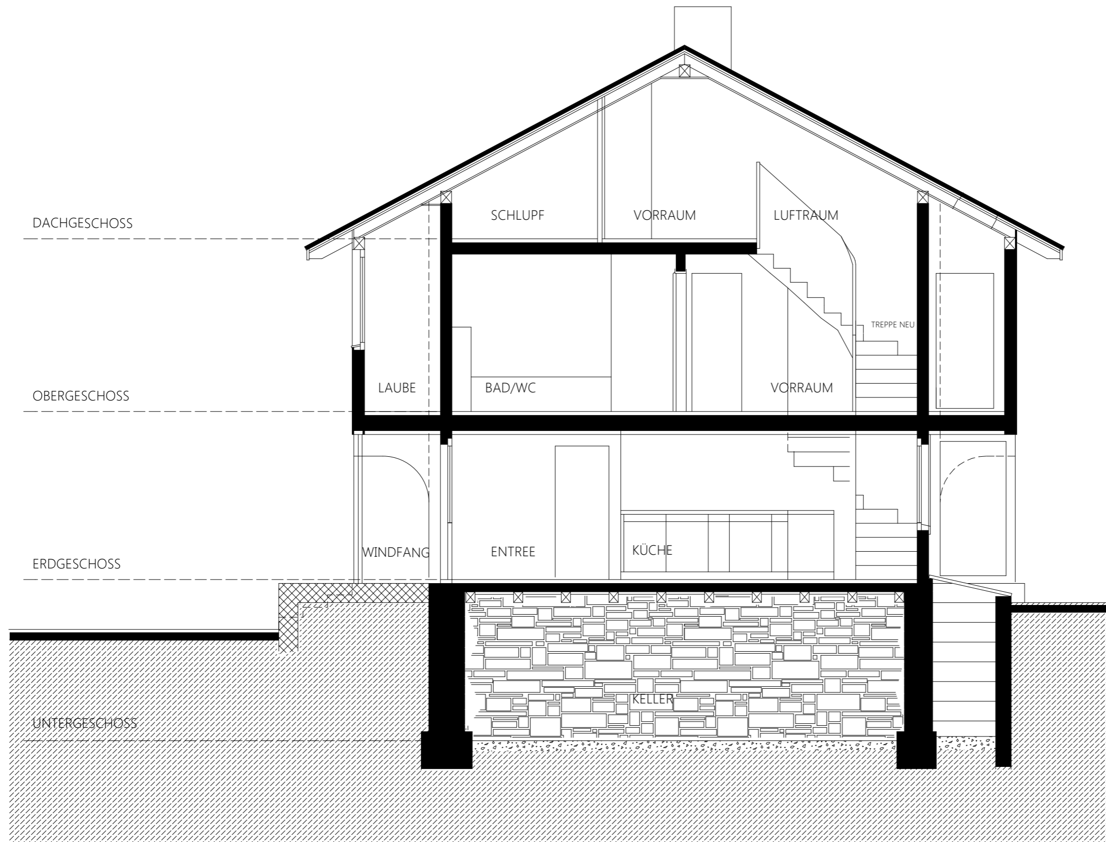
QUERSCHNITT
